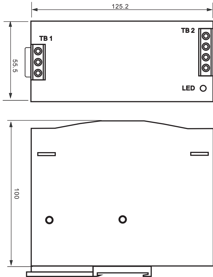
安装导轨: TS35/7.5或TS35/15
